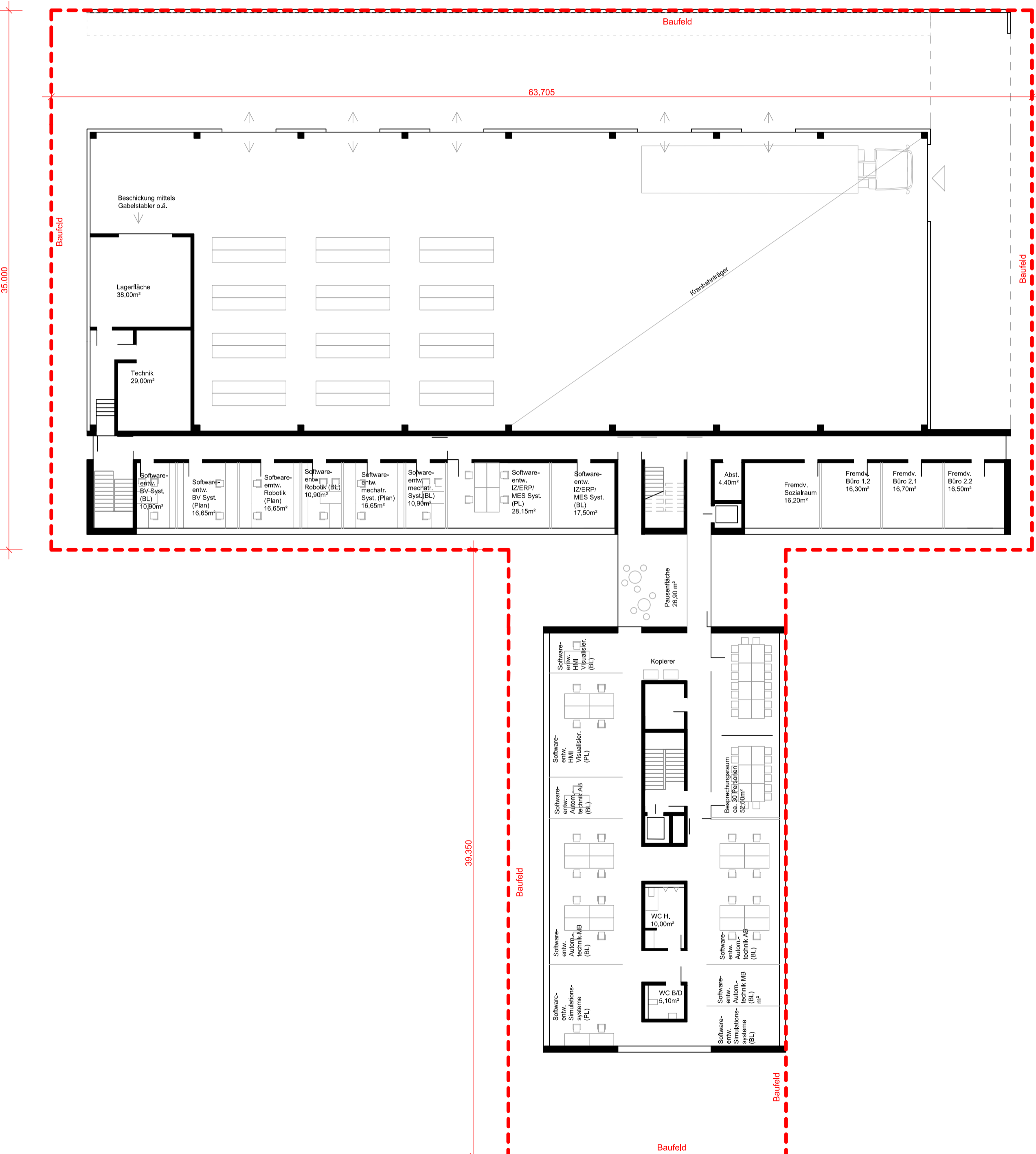
Obergeschoss
